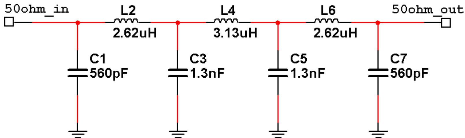
Ejemplo: Filtro Pasa Bajos Chebyshev Banda de 80m con valores normalizados de capacidad
